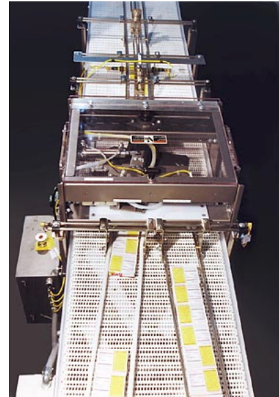
Small Carton 1 : 2 Divert
