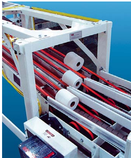
2 : 3 Vertical Switch
